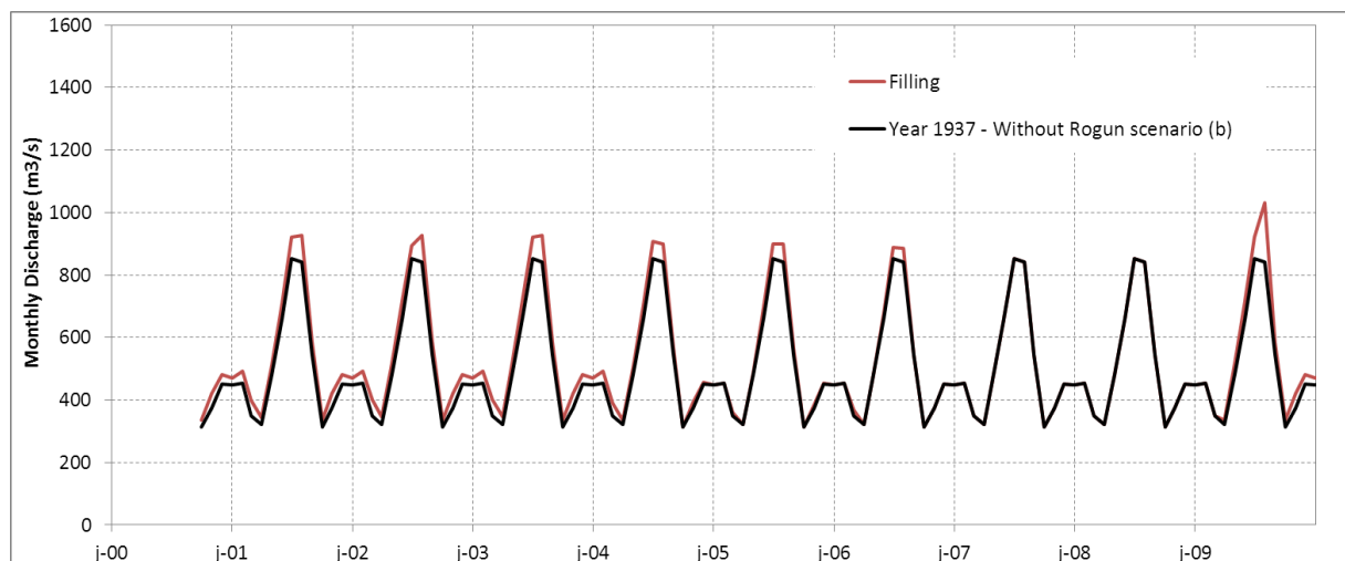
Рисунок 55 : Приток в нижней части р. Вахш – заполнение НПУ – 1220 мнум
