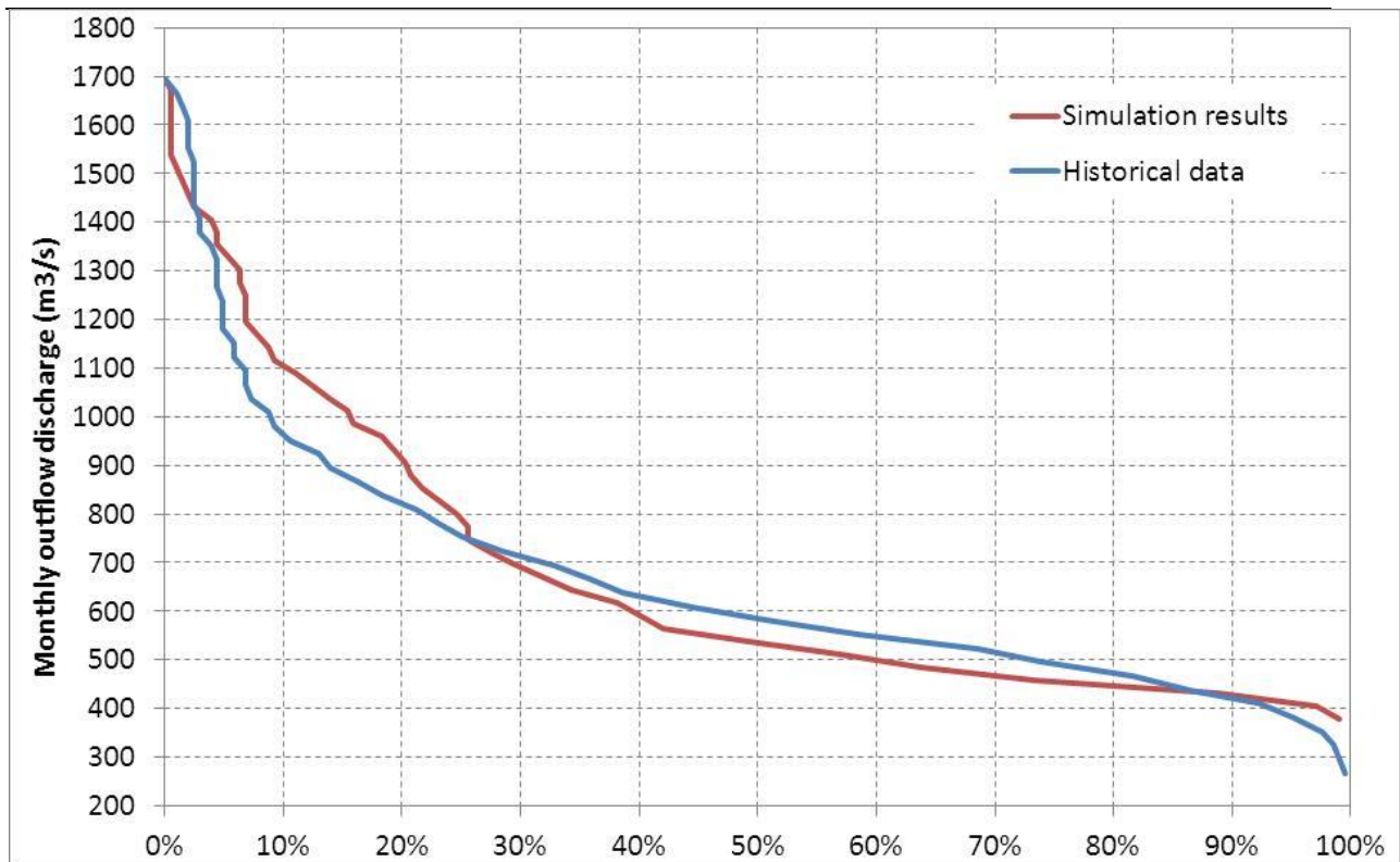
Рисунок 47 : Кривая протяженности оттоков Нурека – Историческая и моделированная)
