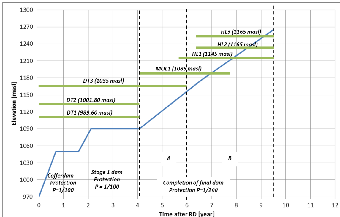
Рисунок 32: НПУ = 1255 м.н.у.м. – Эксплуатационный диапазон сооружений отвода
