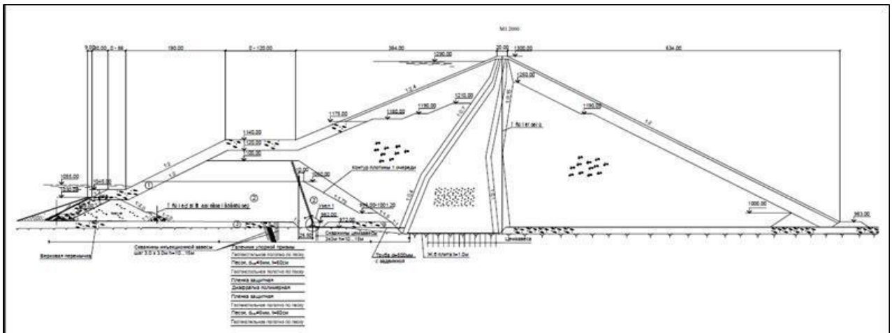
Рисунок 19: Расчет поперечного сечения (Трехмерное моделирование устойчивости плотины, Гидропроект, 2009 год)
