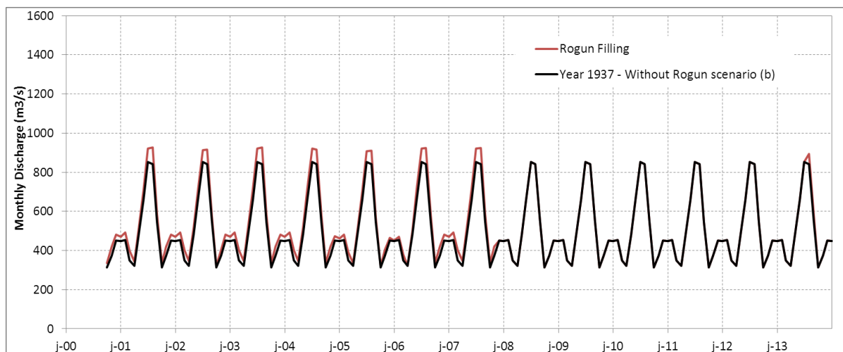
Рисунок 53 : Приток на нижнем конце р. Вахш – Наполнение, НПУ =1255 мнум
