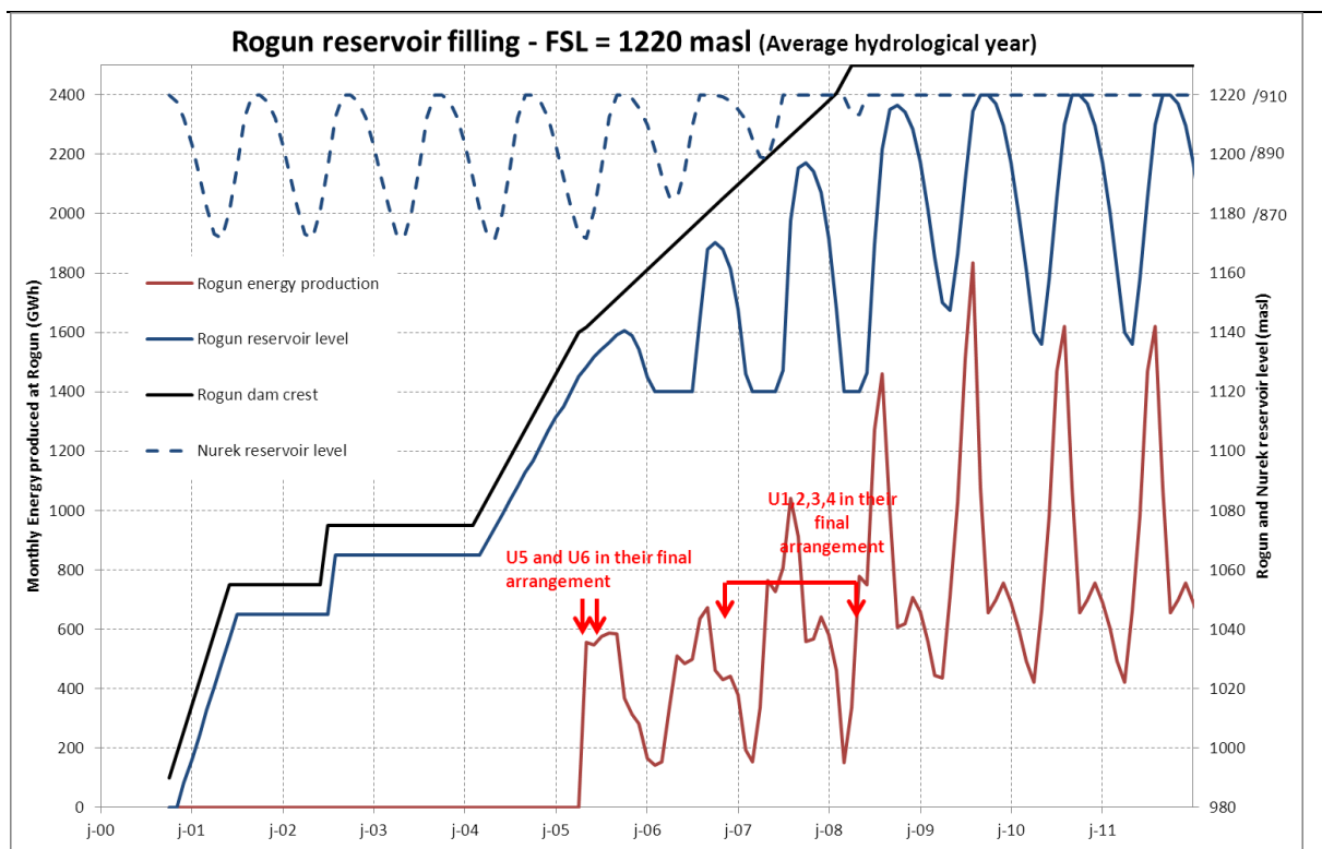
Рисунок 54 : Наполнение водохранилища Рогун - Результаты моделирования, НПУ = 1220 мнум
