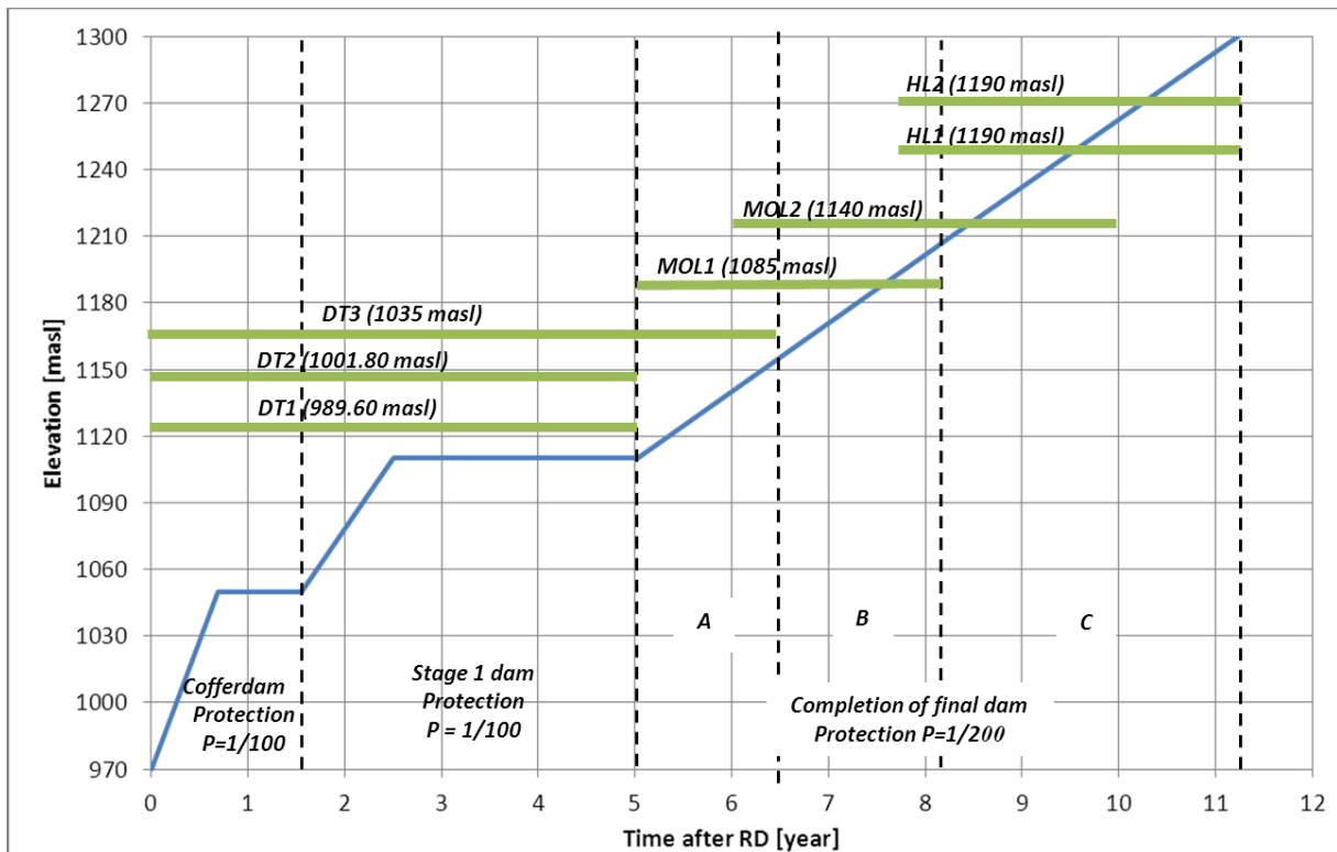
Рисунок 30 : НПУ = 1290 м.н.у.м. – Эксплуатационный диапазон сооружений отвода
