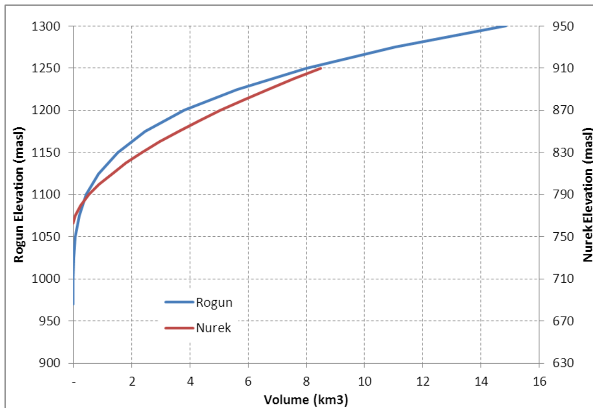
Рисунок 39: Объем водохранилищ Рогун и Нурека относительно отметок
