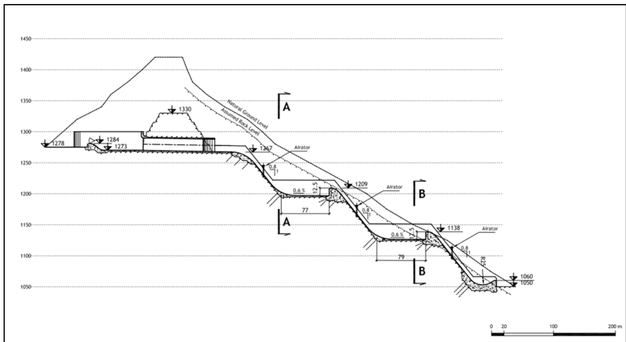
Рисунок 13: Продольное сечение ступенчатого водосброса
