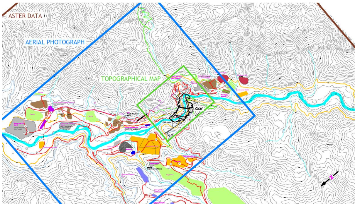
Рисунок 1: Топографические данные
