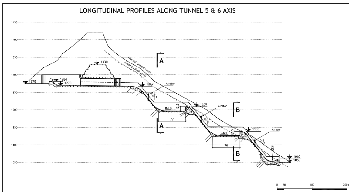
Рисунок 11 : Продольное сечение предложенного поверхностного водосброса
