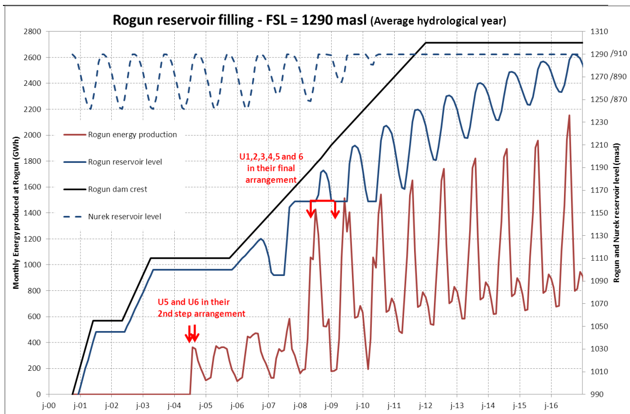
Рисунок 50 : Наполнение водохранилища Рогунской ГЭС - Результаты моделирования НПУ=1290 мнум
