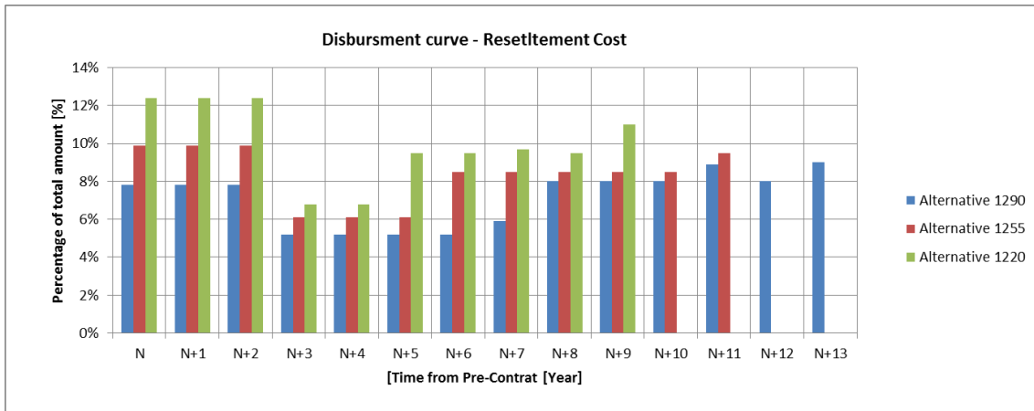
Рисунок 64: Кривая расходов – Затраты на переселения и замены инфраструктуры
