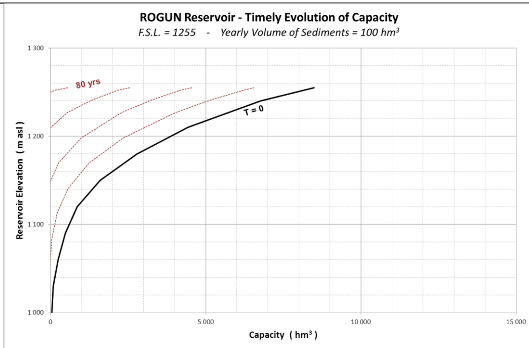
Рисунок 41 : Объем водохранилища Рогуна НПУ =1255 мнум- влияние наносов
