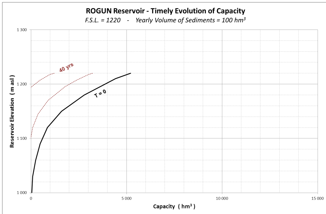
Рисунок 42: Объем водохранилища Рогуна НПУ =1220 мнум- влияние наносов
