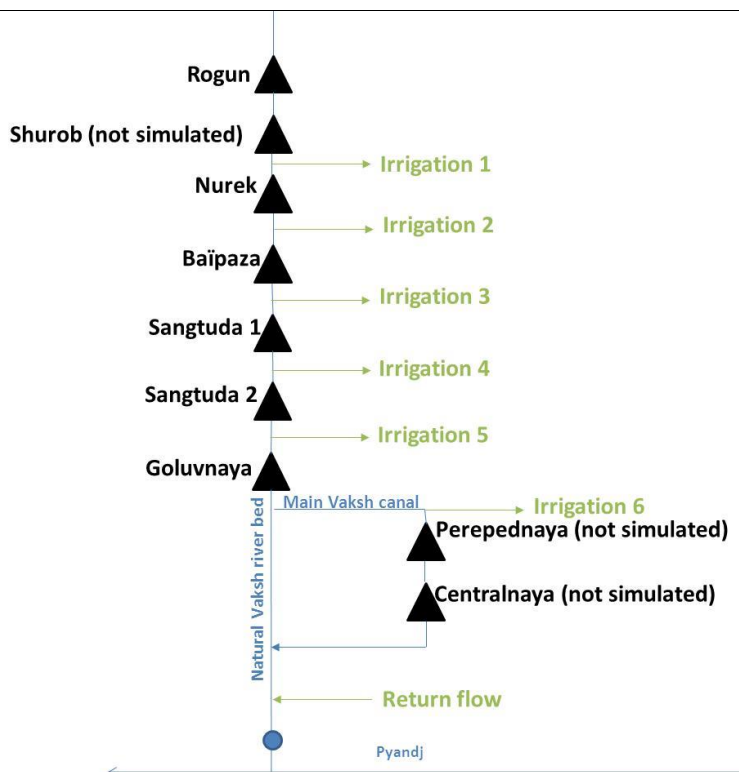
Рисунок 38: Схема Вахшского каскада
