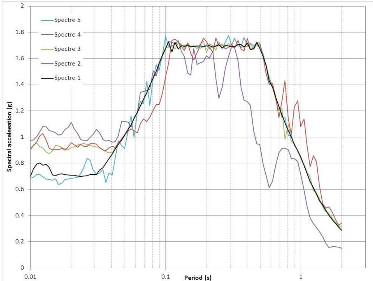
Рисунок 22: Распределение спектрального ускорения MP3 (величина затухания 5%)
